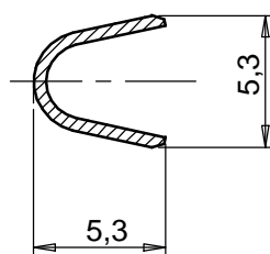
SEZIONE A-A
