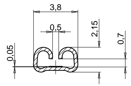
SEZ. A-A
